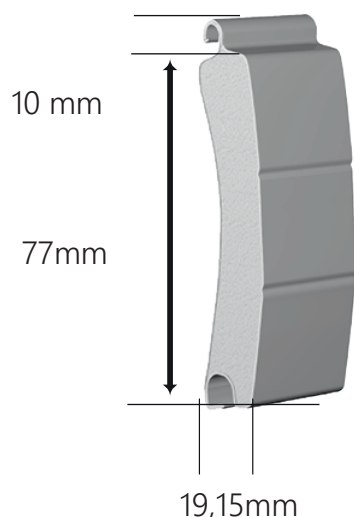
Lame aluminium avec mousse
